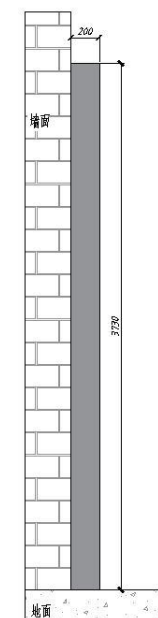
侧视图
