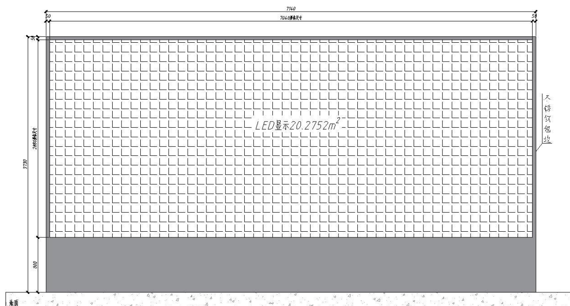
LED显示屏完成面示意图
