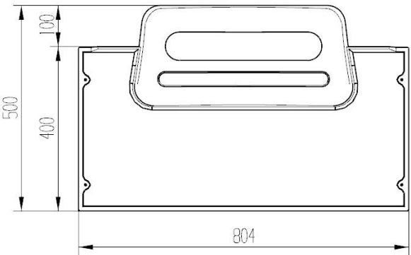
床头安全靠背结构参考图
