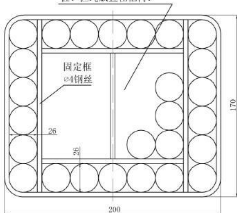
图 C.8 篷杆内包装及固定框主要尺寸
