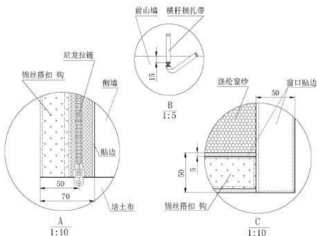
图A.8 篷体侧墙里结构及主要尺寸
