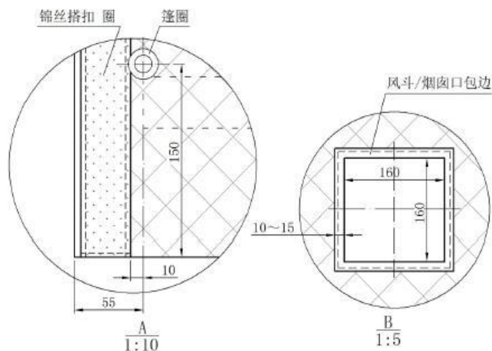
图 A.14 棉内胆无门山墙里结构及主要尺寸
