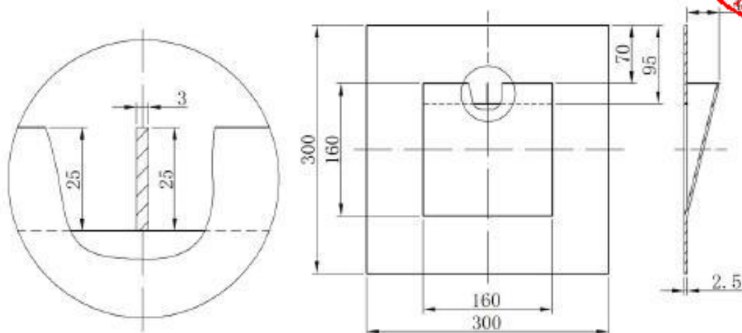
图C.6 风斗结构及主要尺寸
