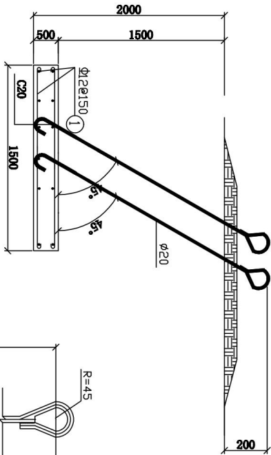
地锚埋设图
