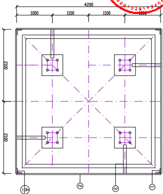
防雷接地平面布置图
