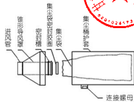
风向跟踪滤袋式沙尘水平通量仪实物图及结构示意图
