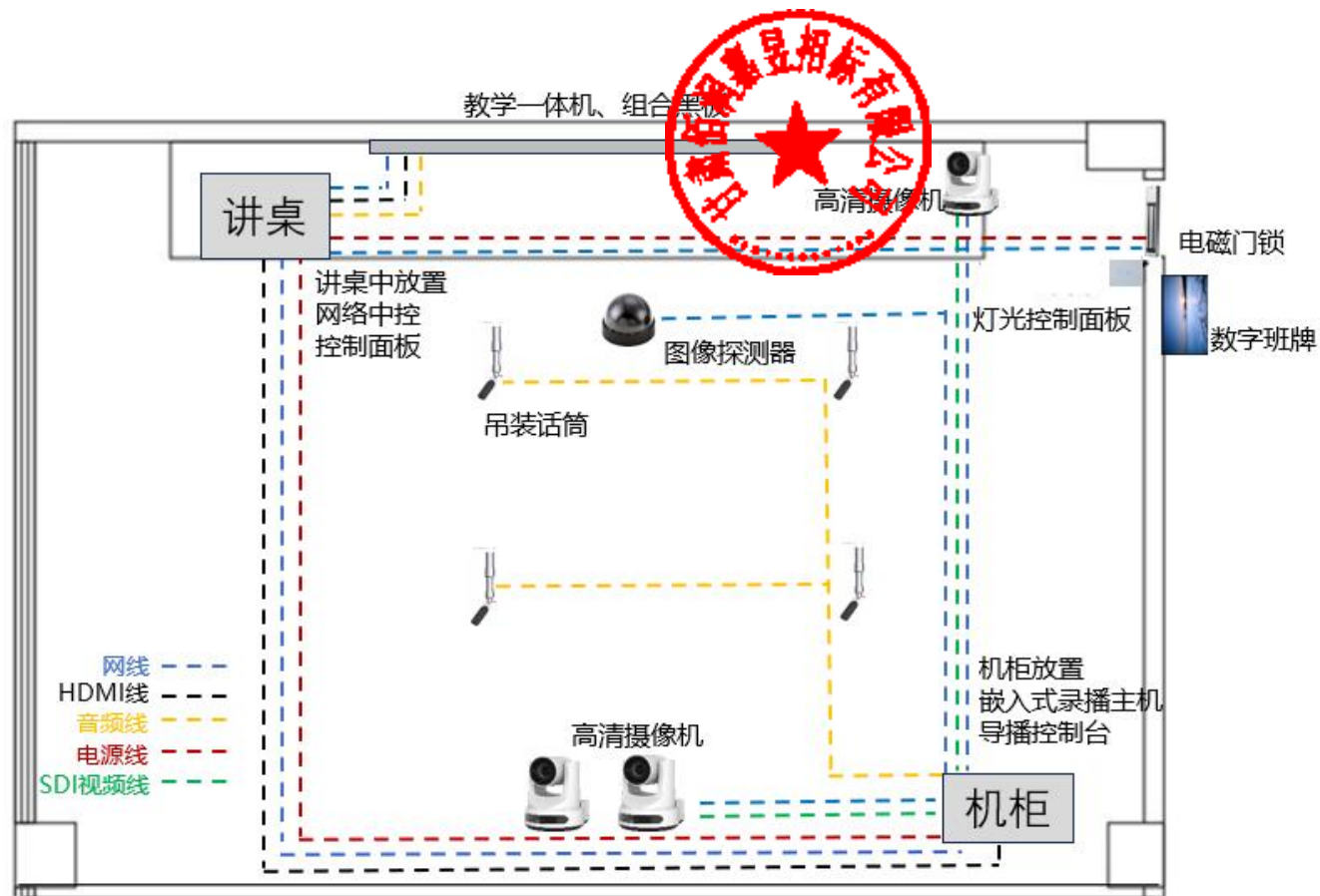
图 7：四号实验楼 5 间微格教室布线图
