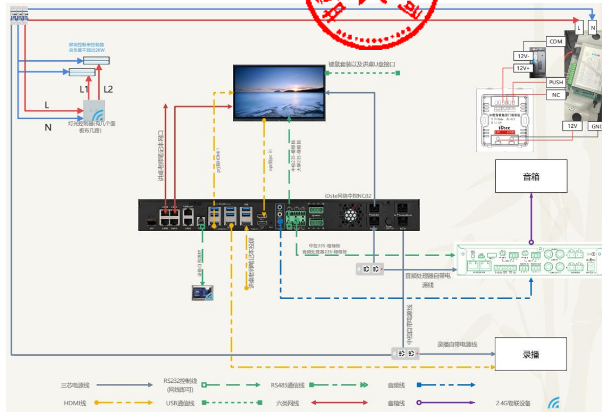
图 10：网络中控连线图
