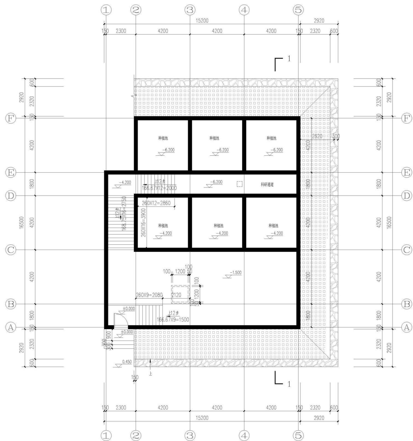
一层平面图 1:100
