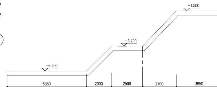
1-1 1:100
