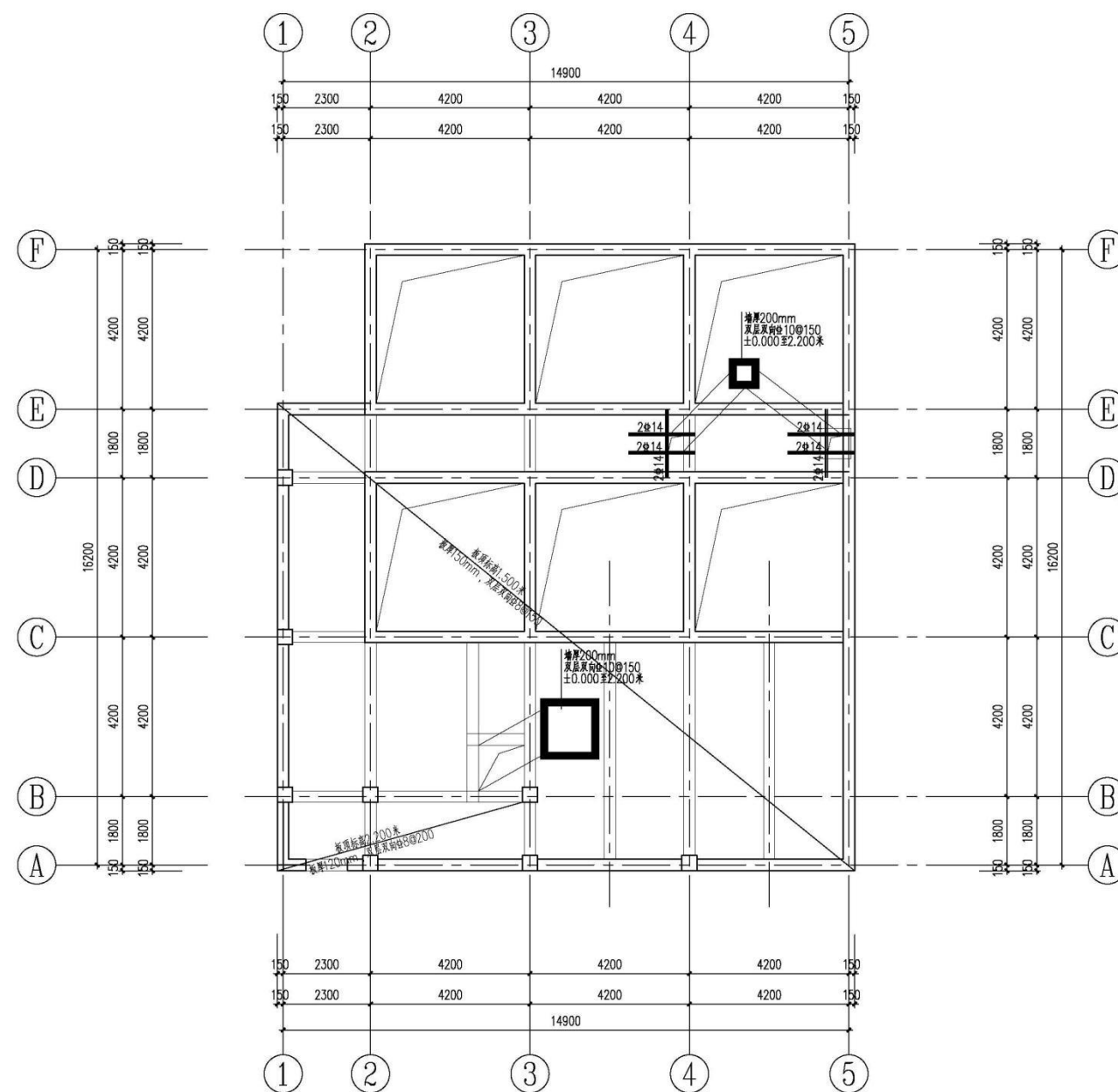
标高1.500米板平面图 1:100
