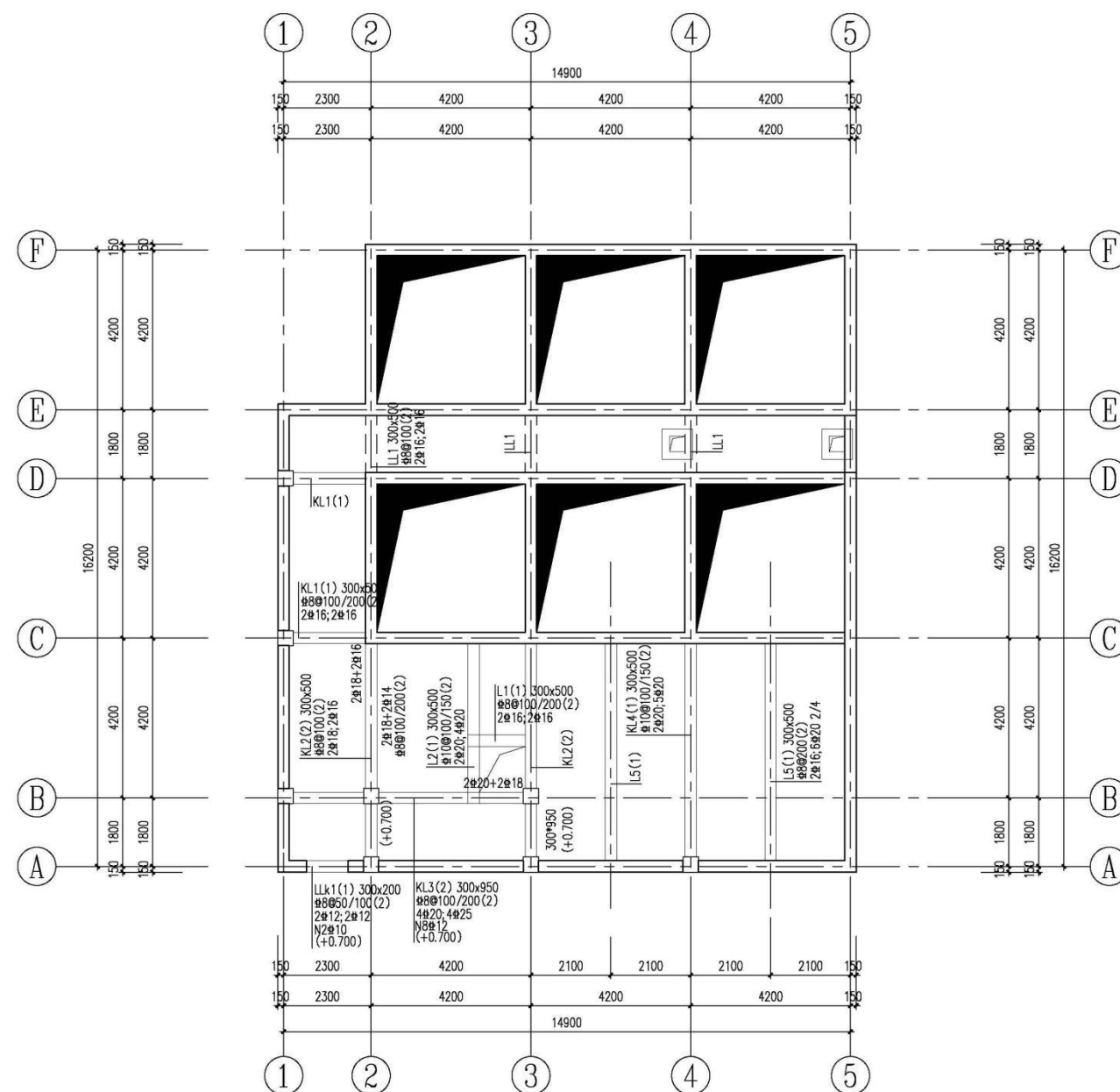
标高1.500米梁平面图 1:100
