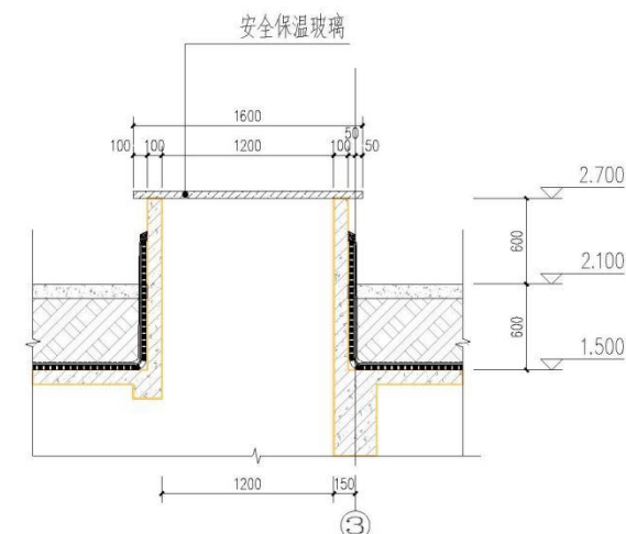
1 1:50
