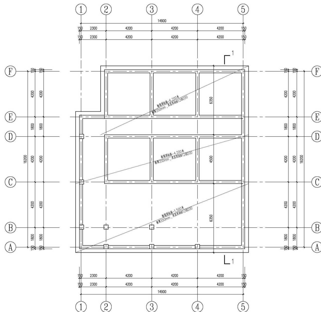
基础平面图 1:100
