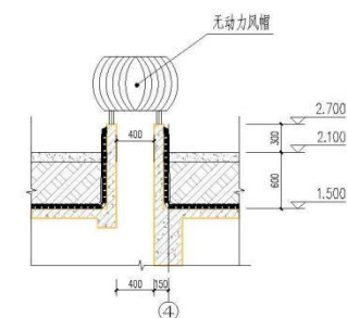
2 1:50
