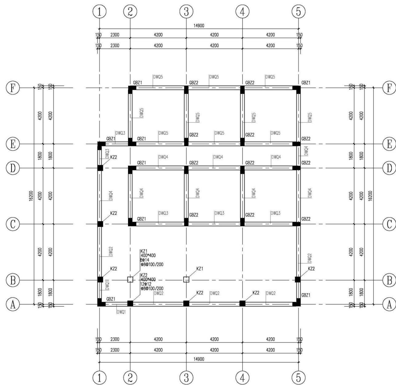
基础顶至±0.000墙柱平面图 1:100
