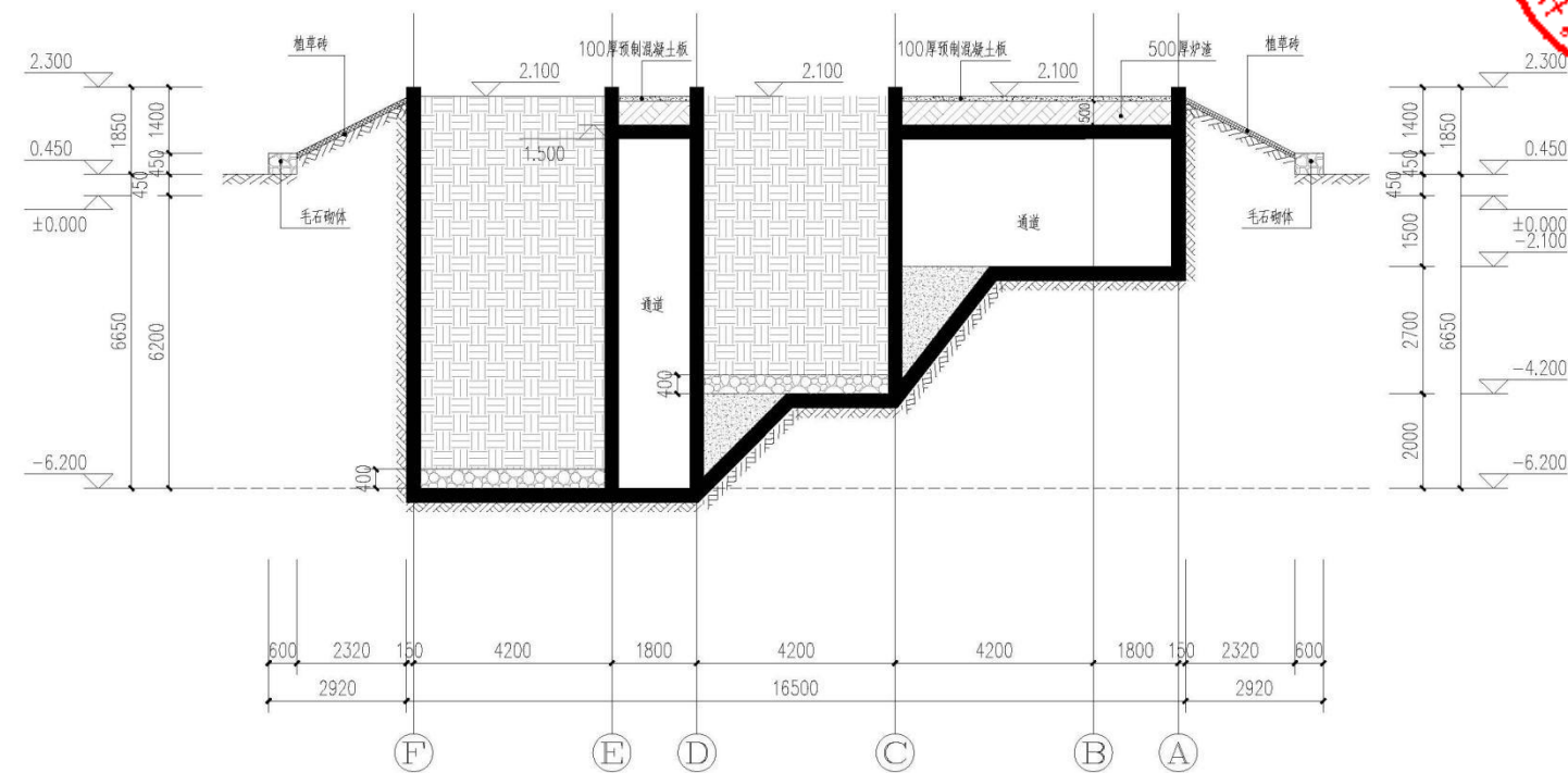
1-1剖面图 1:100
