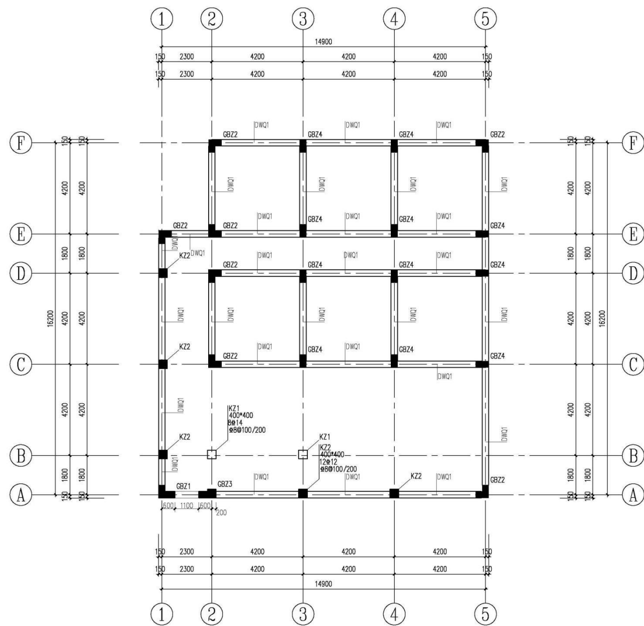
±0.000至2.200墙柱平面图 1:100
