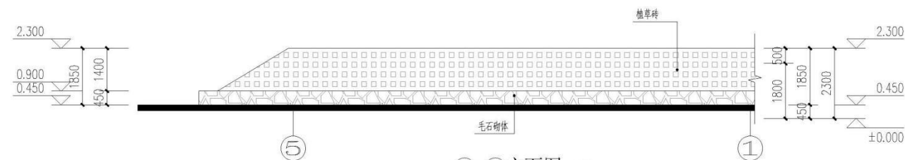
6-1立面图 1:100
