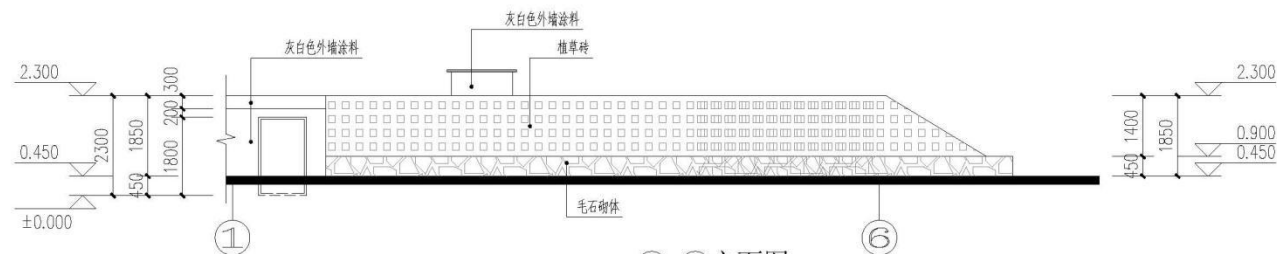
1-6立面图 1:100
