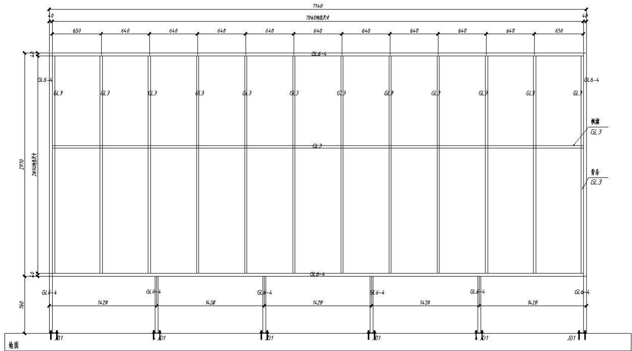
结构正立面图
