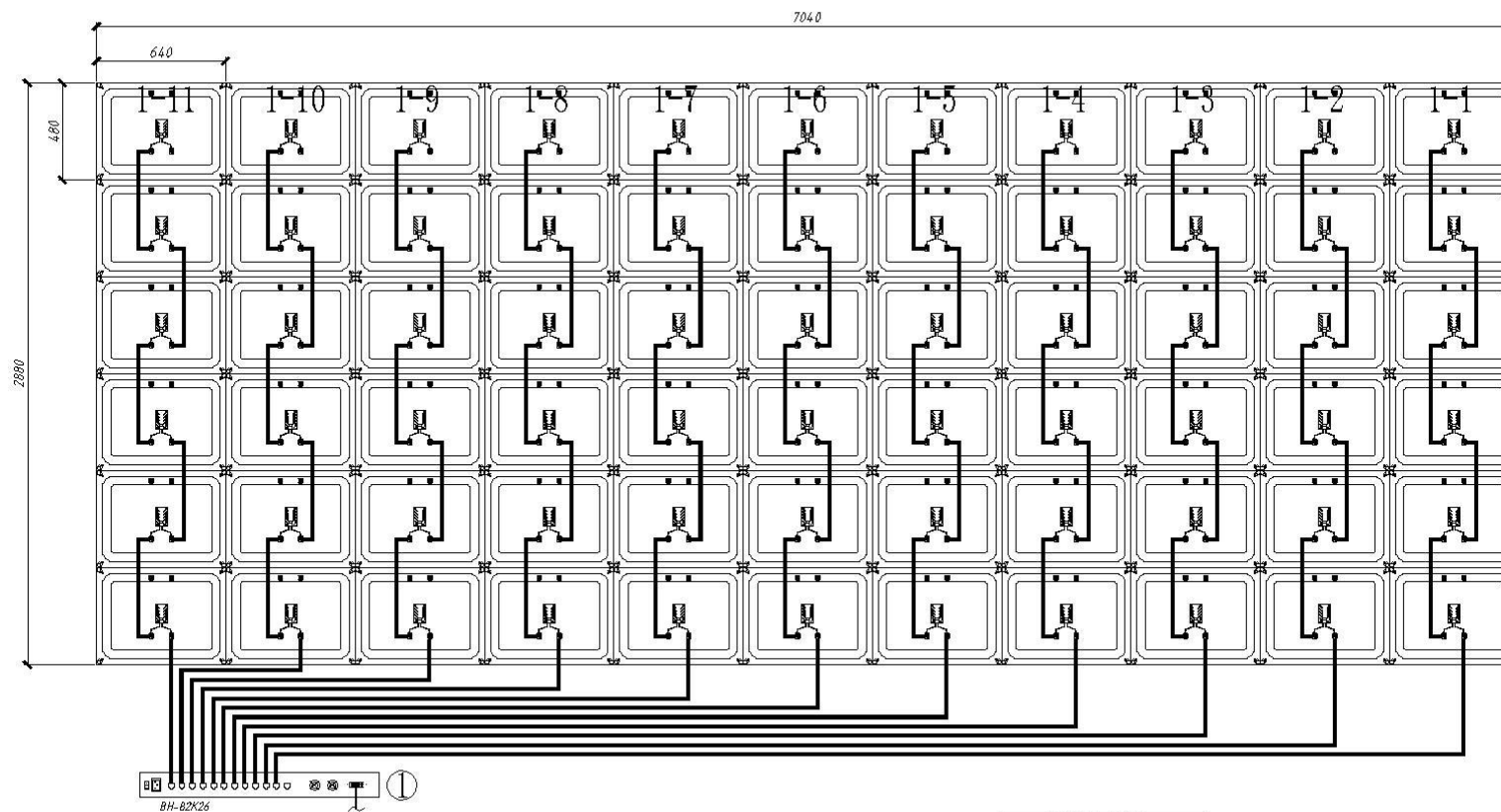
信号连接示意图 (从屏体背面看)
