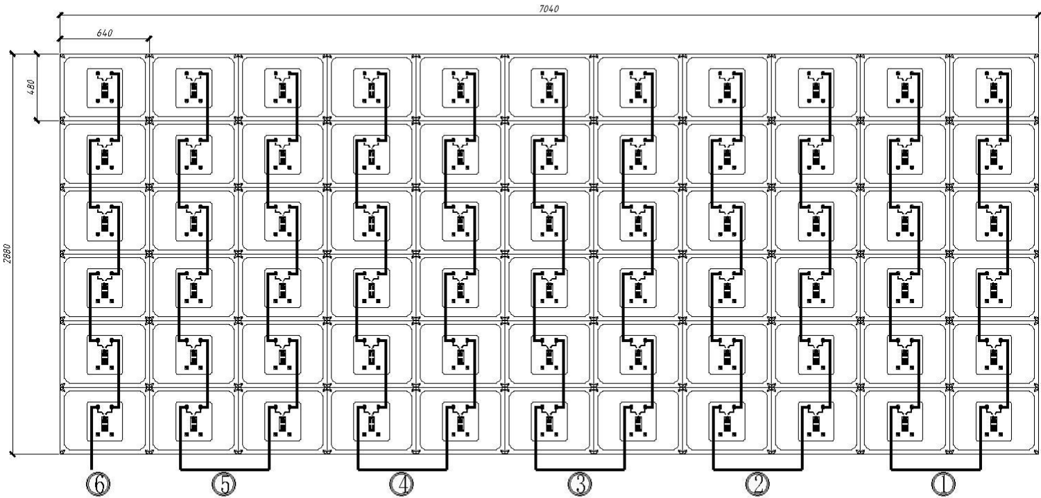
强电连接示意图 (从屏体背面看)
