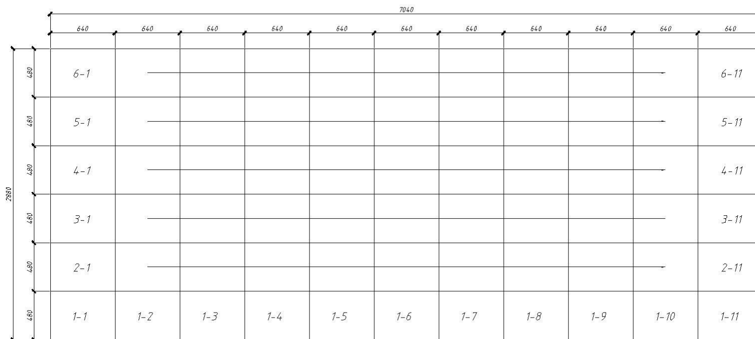
箱体排布图 (从屏体背面看)
