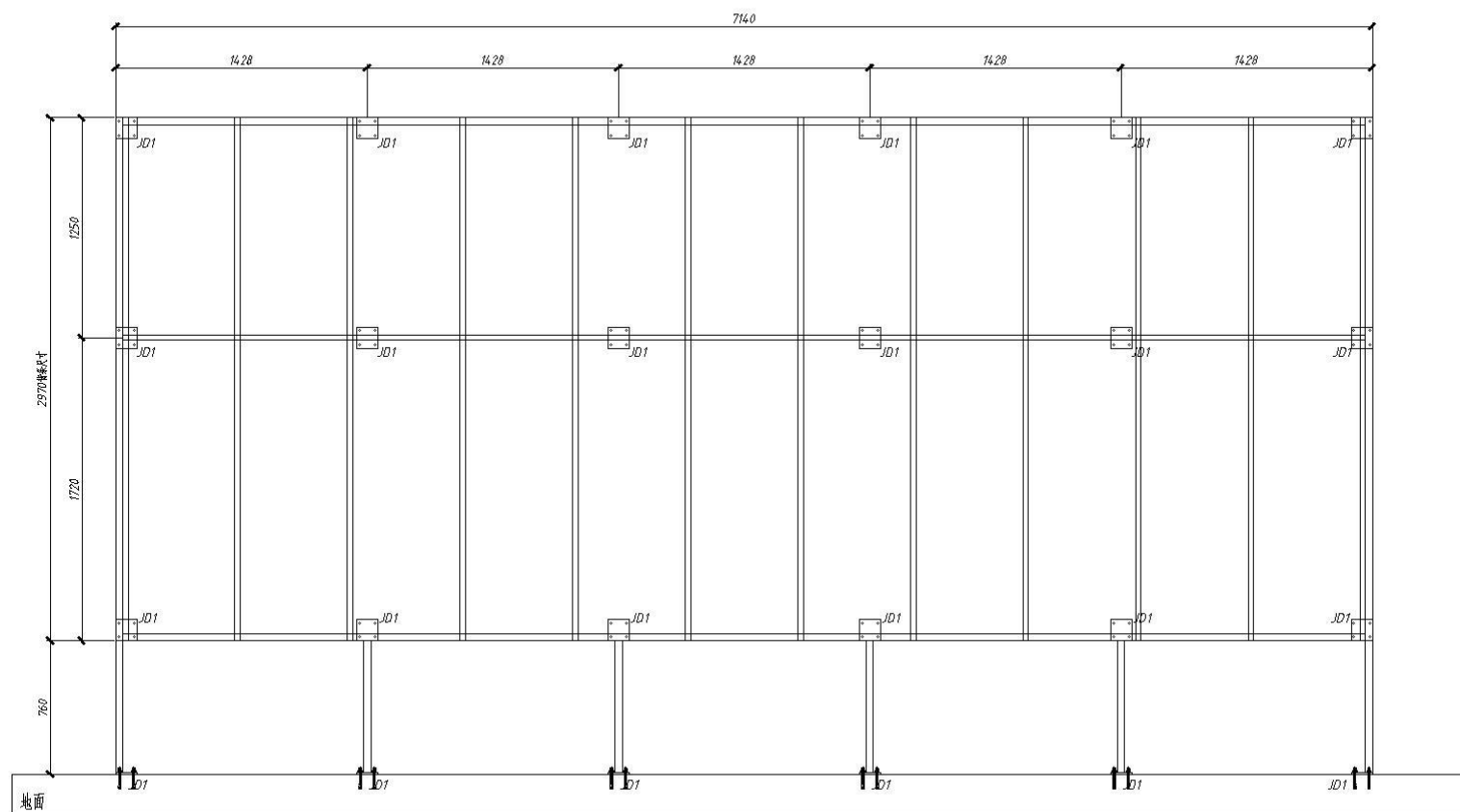
结构正立面图
