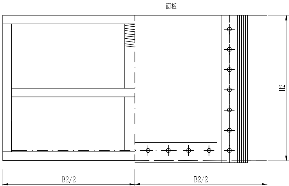
闸门板设计图
