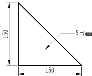
腹板大样图
