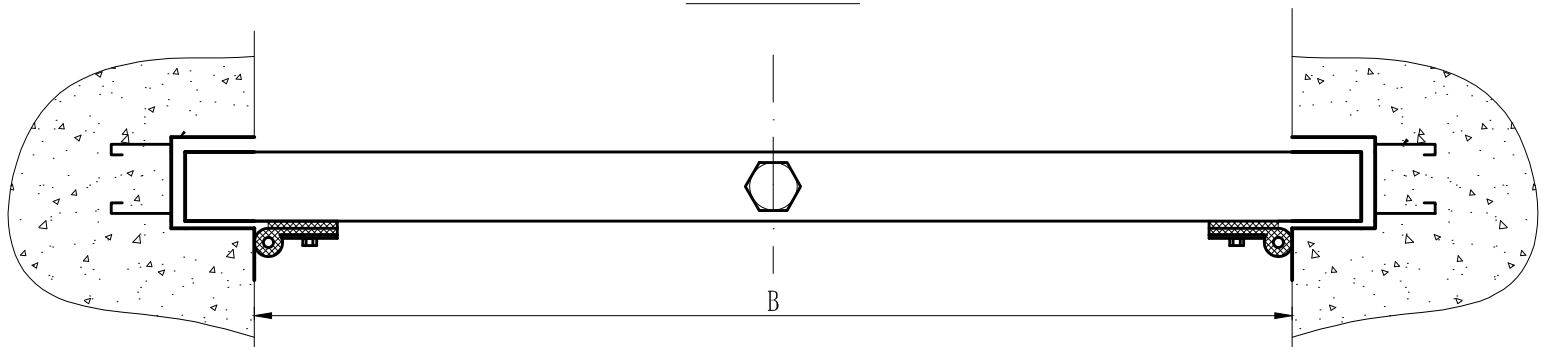
闸门剖面图
