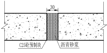
伸缩缝大样图
