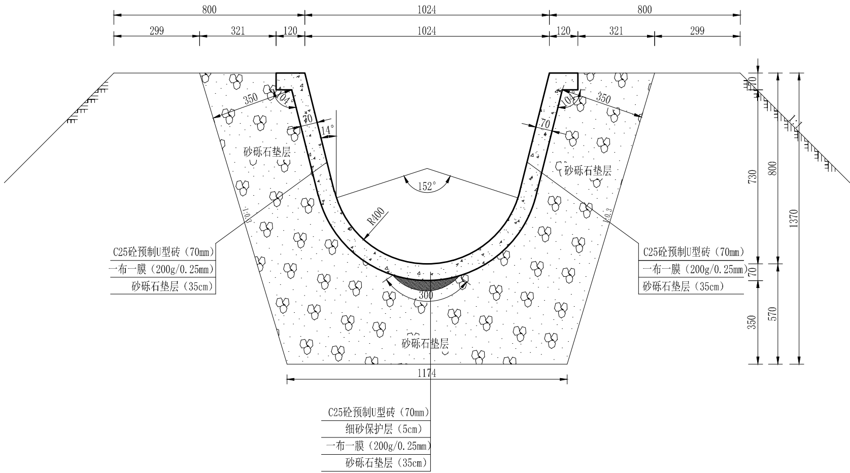
U80渠道横断面图
