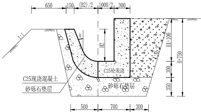
渐变段剖面图
