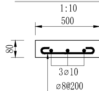
人行桥板配筋图
