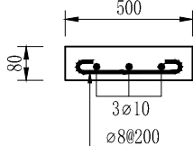
人行桥板配筋图
