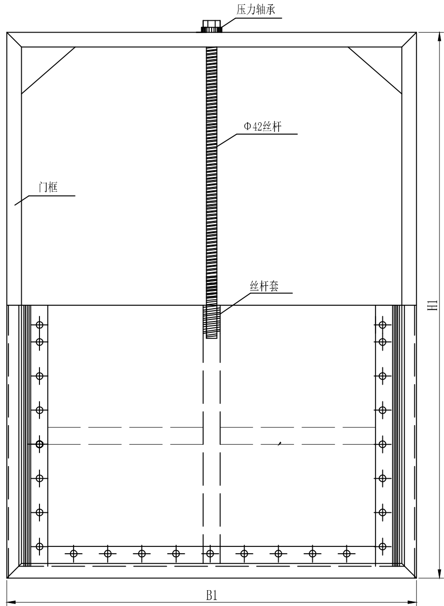
钢闸门设计图
