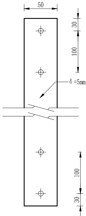
压条大样图
