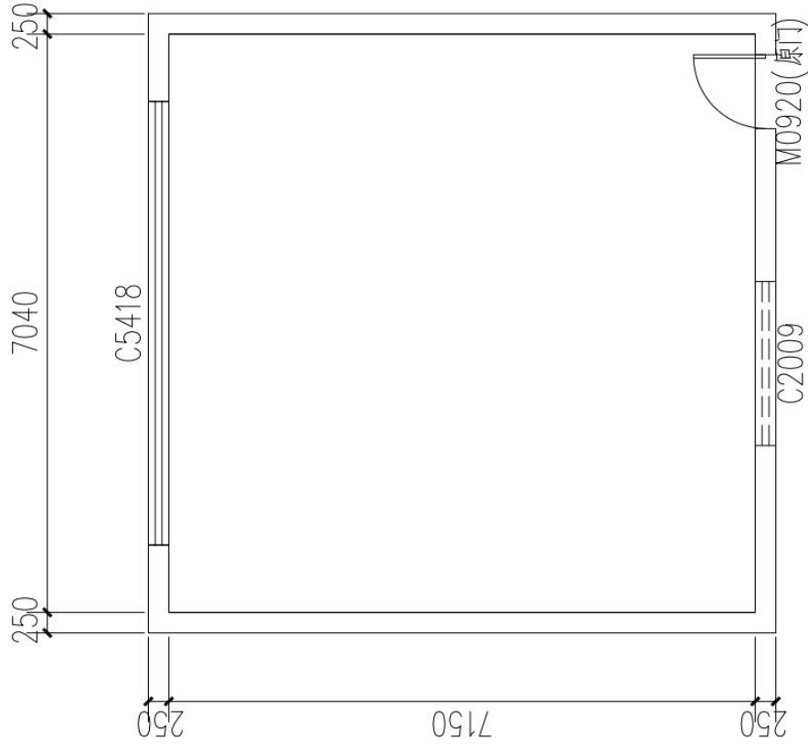
(504) 原平面图 1:100
