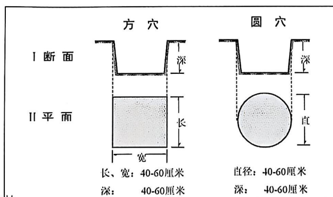
穴状整地断面、平面图
