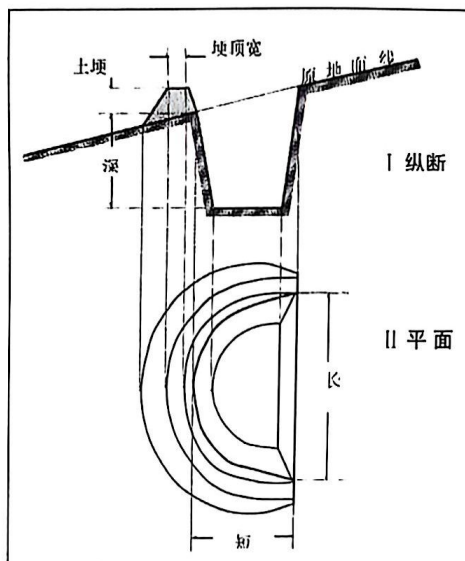
鱼鳞坑整地纵断面、平面图
